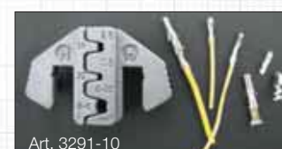
Art. 3291-10 DIN 2.5 / 0.5 / 8-10 mm 2 AWG 14 / 22 / 8-6
